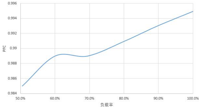
KVG-12500-DH PFC曲线
