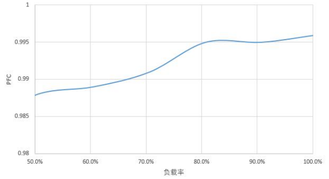
KVG-24600-DH PFC曲线
